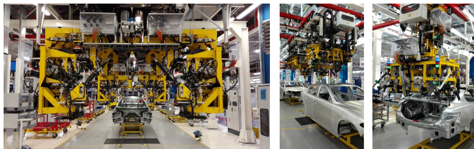
LINEA DI FERRATURA 949-952 CASSINO
