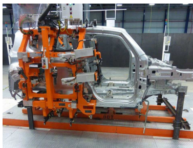
LINEA DI FERRATURA 949-952 CASSINO
