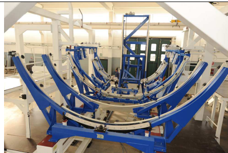
ATTREZZI DI GRAFFATURA (ROLLER HEMMING e TABLE TOP)
