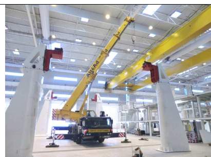
ATTREZZI ASSEMBLAGGIO PANNELLI LATERALI A350
